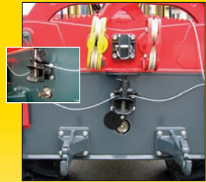
Dreipunkteinrichtung mit Zapfwellenabtrieb
